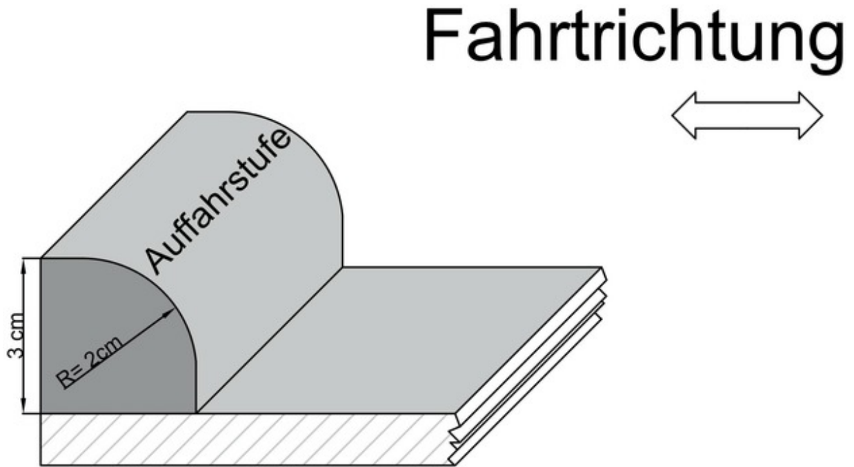
Bild 4: Bordsteinprofil
