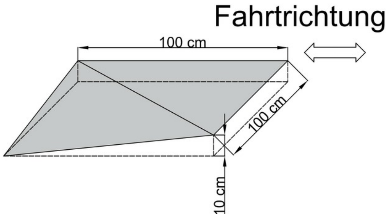
Bild 3: Einseitige Absenkung
